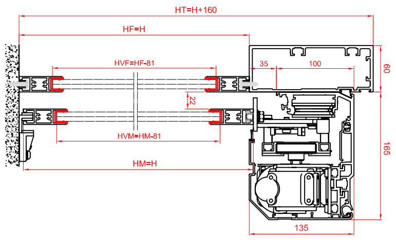
Section Scale: 1/2
