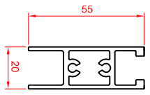
Section Scale: 1/2
