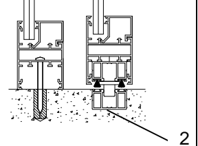
Guía empotrada
