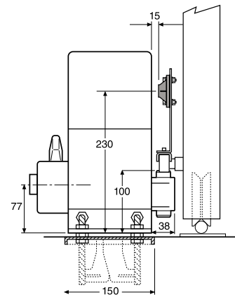
Cotas de montaje
