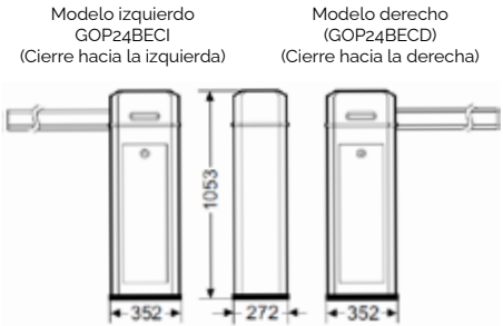
Cuerpo de acero S235 lacado.
